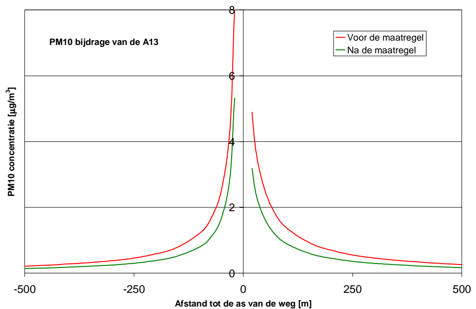
Figuur 8 De verminderde bijdrage van de A13 aan de jaargemiddelde concentratie van PM10 als gevolg van de 80 km/u maatregel in Overschie tot 500 m ten westen en oosten van de A13.
